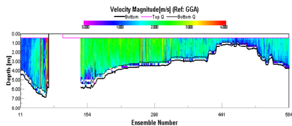
図-1 データ欠測が多いADCP流況観測事例 6)
