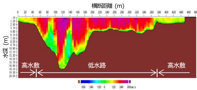
(b) 流下軸方向の流速分布 ( Q=5095\text{m}^3/\text{s} )
